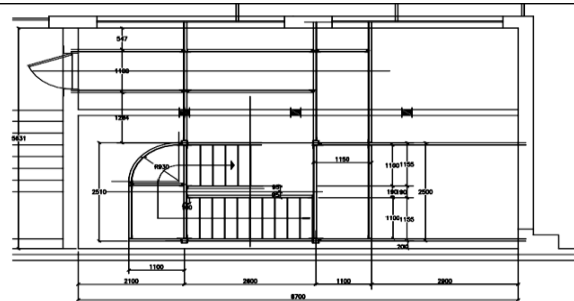
PLANTA NIVEL +1130
