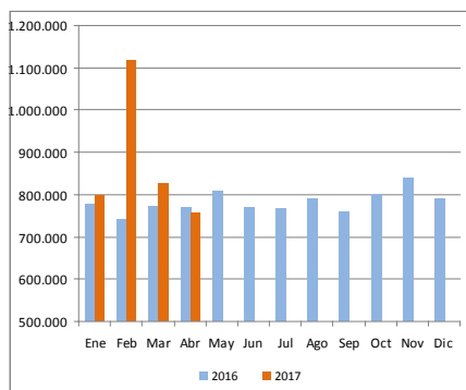
Gráfico 1. Energía autogenerada total en MW/h
