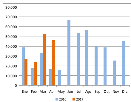
Gráfico 6. Energía cogenerada para autoconsumo en MW/h
