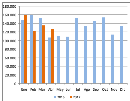
Gráfico 5. Energía cogenerada despachada al MEM en MW/h
