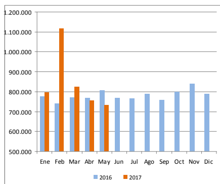
Gráfico 1. Energía autogenerada total en MW/h
