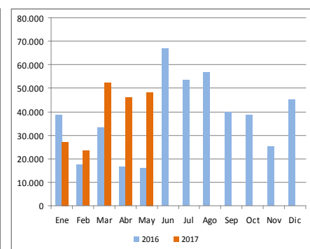
Gráfico 6. Energía cogenerada para autoconsumo en MW/h
