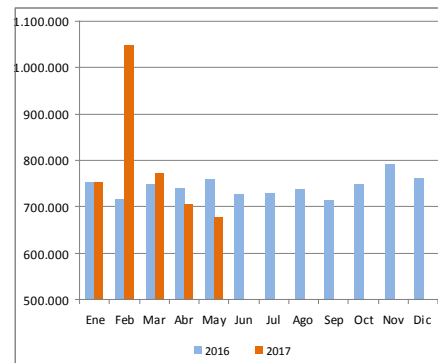
Gráfico 3. Energía autogenerada para autoconsumo en MW/h
