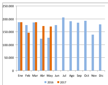
Gráfico 4. Energía cogenerada total en MW/h
