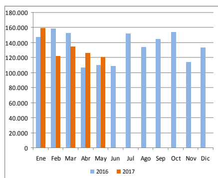
Gráfico 5. Energía cogenerada despachada al MEM en MW/h
