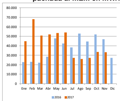
Gráfico 2. Energía autogenerada despachada al MEM en MW/h
