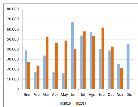
Gráfico 6. Energía cogenerada para autoconsumo en MW/h
