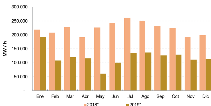
Gráfico 2.4 Energía cogenerada total en MW/h. Industria manufacturera. Enero 2018-diciembre 2019
