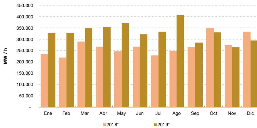
Energía autogenerada despachada al MEM en MW/h. Minería e industria manufacturera. Enero 2018-diciembre 2019
