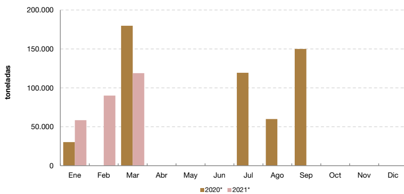
Gráfico 3.3 Exportaciones de biodiésel, en toneladas. Enero 2020-marzo 2021
