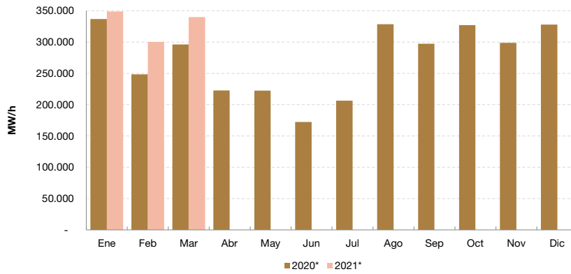
Energía autogenerada despachada al MEM en MW/h. Minería e industria manufacturera. Enero 2020-marzo 2021
