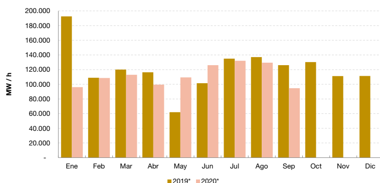
Gráfico 2.4 Energía cogenerada total en MW/h. Industria manufacturera. Enero 2019-septiembre 2020
