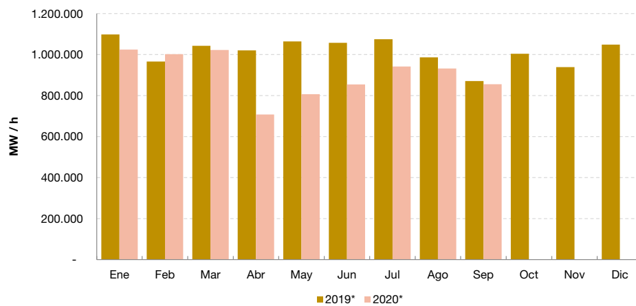
Energía autogenerada para autoconsumo en MW/h. Minería e industria manufacturera. Enero 2019-septiembre 2020
