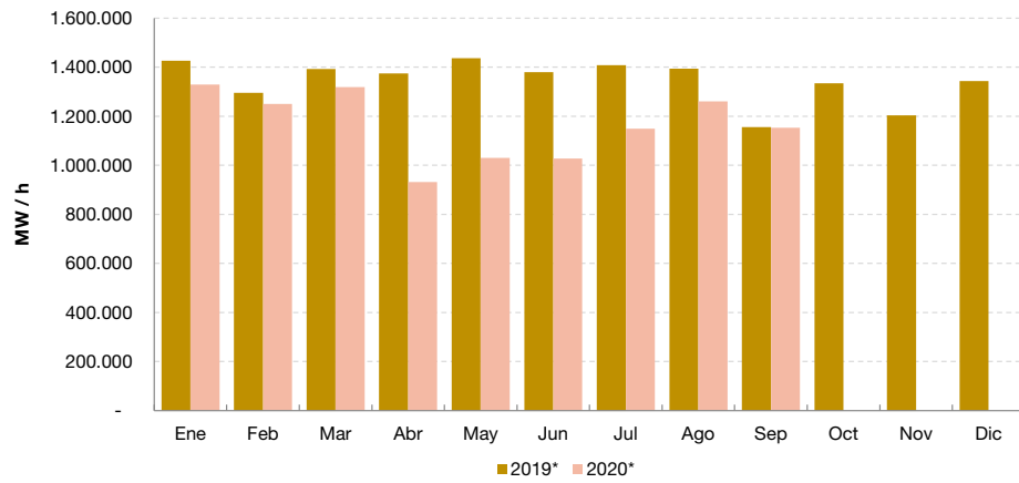
Energía autogenerada total en MW/h. Minería e industria manufacturera. Enero 2019-septiembre 2020
