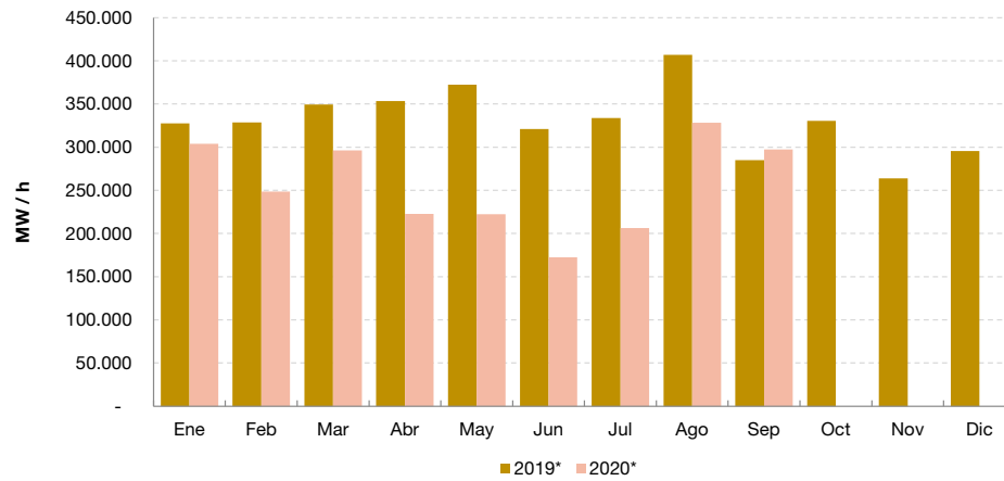
Energía autogenerada despachada al MEM en MW/h. Minería e industria manufacturera. Enero 2019-septiembre 2020
