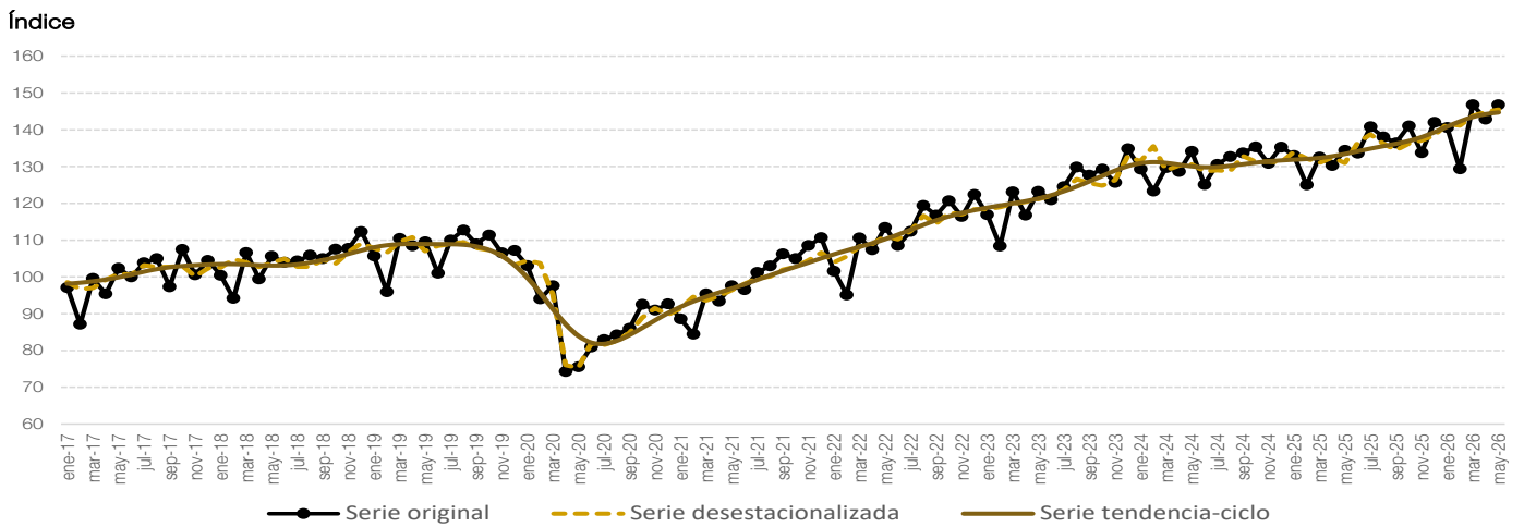
Gráfico 1.1 IPI minero nivel general. Serie original, desestacionalizada y tendencia-ciclo, base 2016=100, en números índice. Enero 2017-mayo 2026
