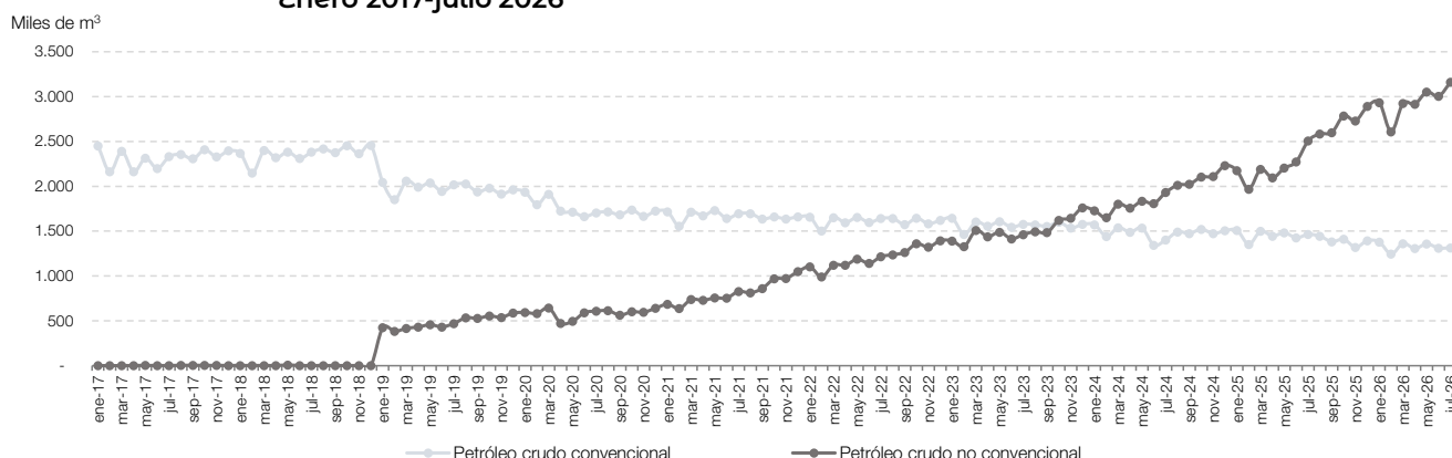
Gráfico 6.2 Extracción de petróleo crudo convencional y no convencional, en miles de m 3 . Enero 2017-julio 2026
