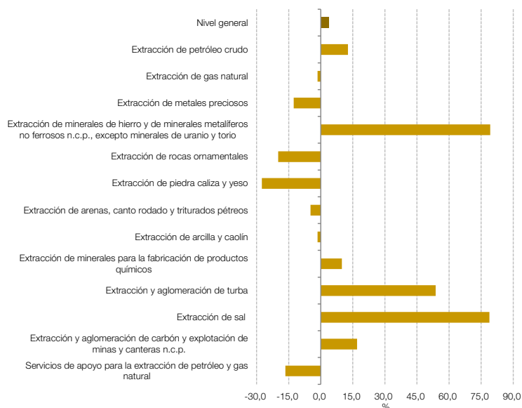
Gráfico 5.1 IPI minero nivel general y subclases, variación porcentual interanual. Julio de 2026
