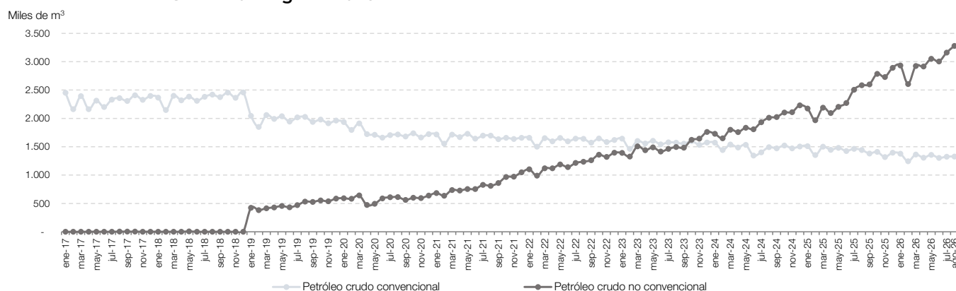
Gráfico 6.2 Extracción de petróleo crudo convencional y no convencional, en miles de m 3 . Enero 2017-agosto 2026
