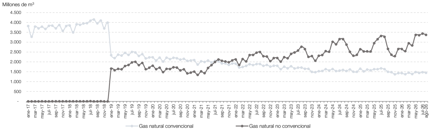
Gráfico 7.2 Extracción de gas natural convencional y no convencional, en millones de m³. Enero 2017-agosto 2026
