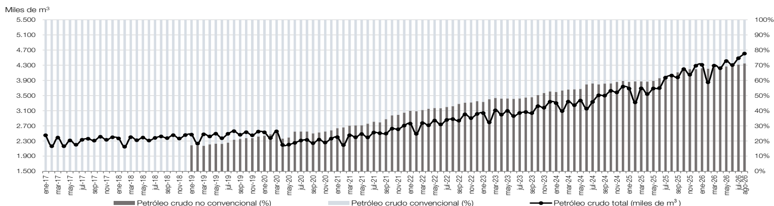
Gráfico 6.1 Extracción de petróleo crudo convencional y no convencional, en miles de m 3 y estructura porcentual. Enero 2017-agosto 2026
