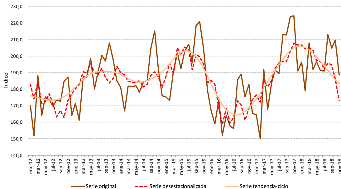
Gráfico 1. Indicador sintético de la actividad de la construcción (ISAC). Serie original, desestacionalizada y tendencia-ciclo, base 2004=100, en números índice. Enero 2012-noviembre 2018
