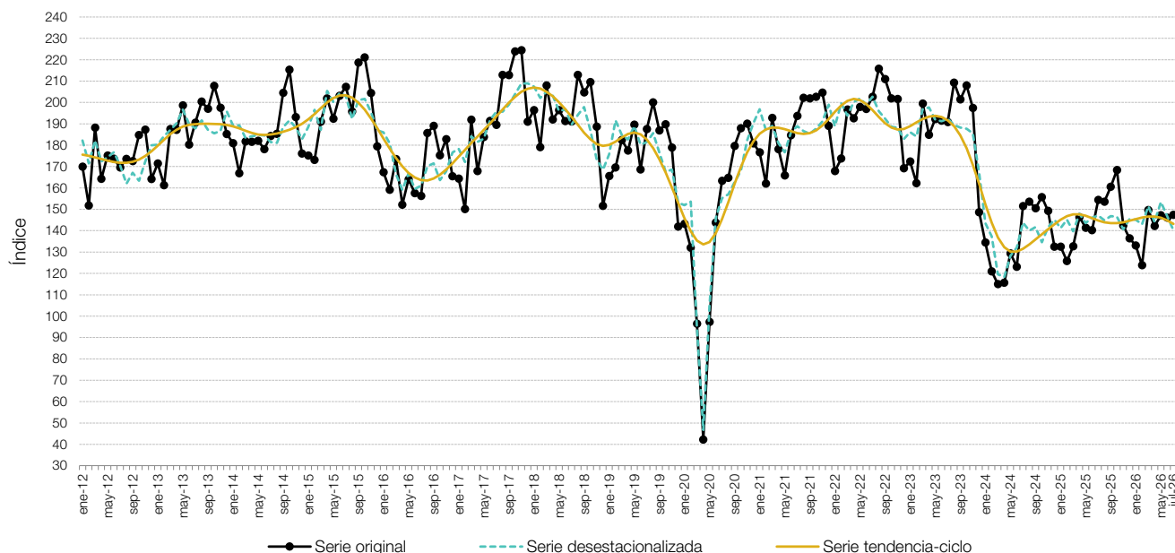
Gráfico 1. Indicador sintético de la actividad de la construcción (ISAC). Serie original, desestacionalizada y tendencia-ciclo, base 2004=100, en números índice. Enero 2012-julio 2026
