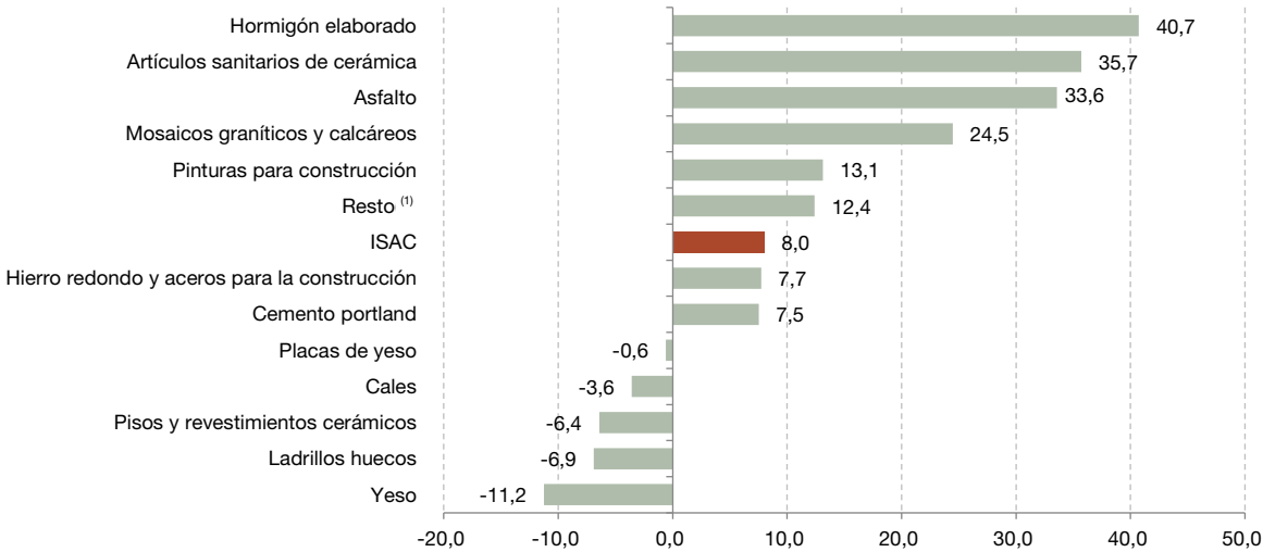
Gráfico 2. Insumos para la construcción. Serie original base 2004=100, en variación porcentual interanual. Octubre de 2025
