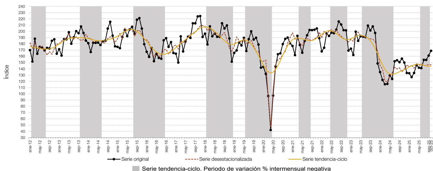
Gráfico 1. Indicador sintético de la actividad de la construcción (ISAC). Serie original, desestacionalizada y tendencia-ciclo, base 2004=100, en números índice. Enero 2012-octubre 2025
